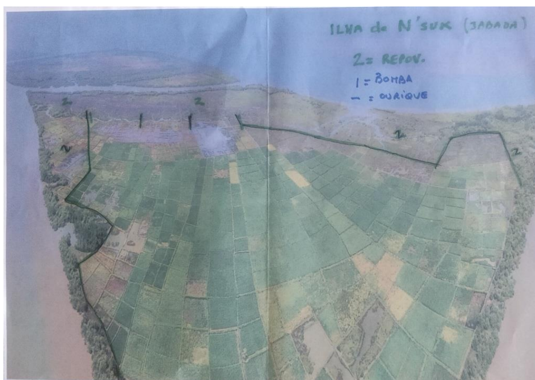
Exemple de priorités de réhabilitation (rizière de Nsuk, village de Jabada Porto) indiquant l'emplacement des digues de ceinture à rehausser et des tubes de drainage à installer.
